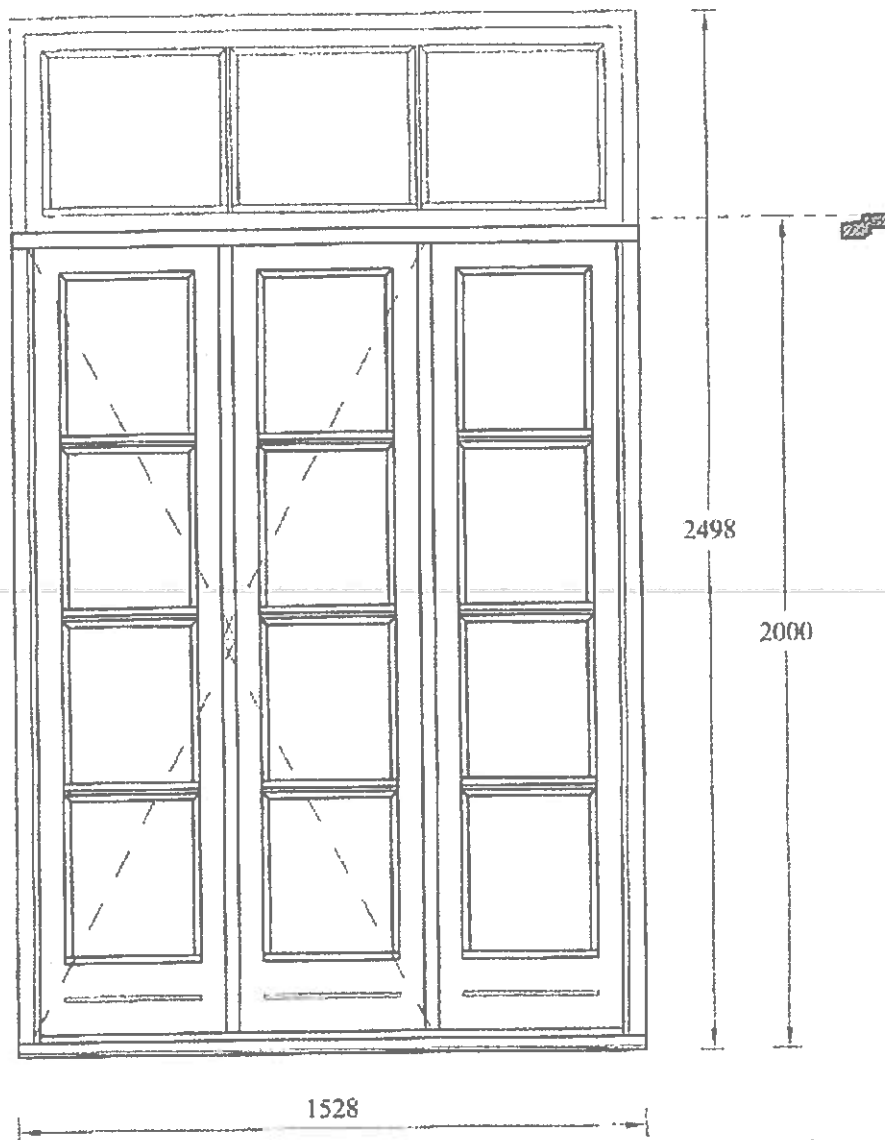
Tegning 1:15
